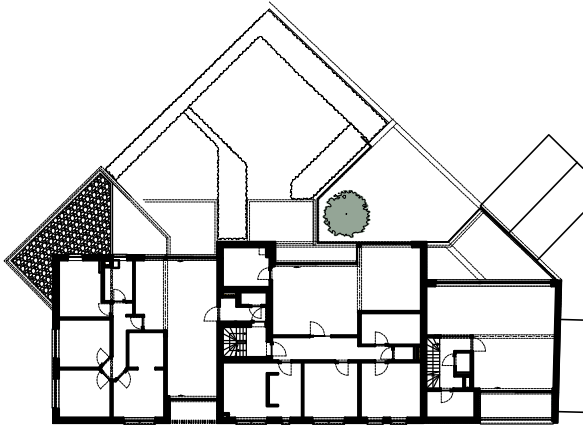
NIVEAU +01
